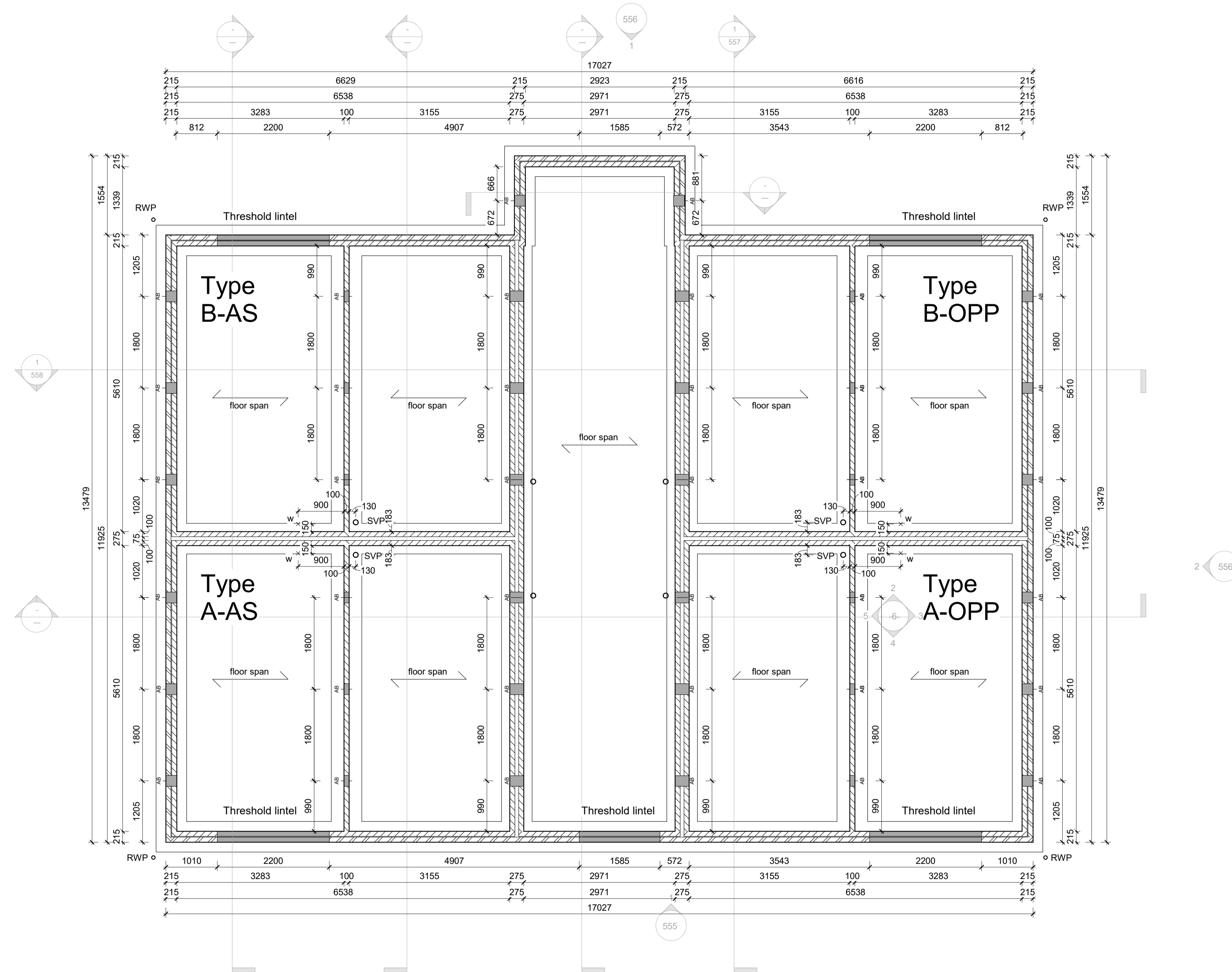
01 Substructure Plan 1 : 50
